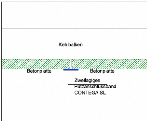
Detail 4 M. 1 : 10
