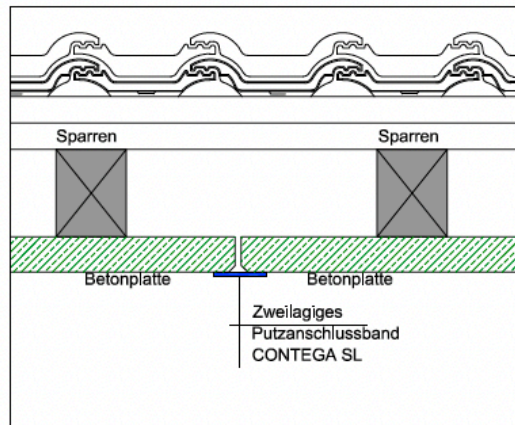
Detail 4 A M. 1 : 10
