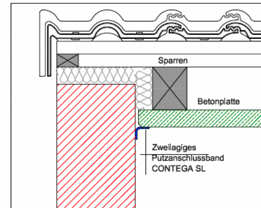
Detail 6 M. 1 : 10
