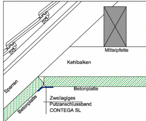
Detail 2 M. 1 : 10
