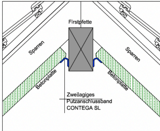
Detail 1 M. 1 : 10
