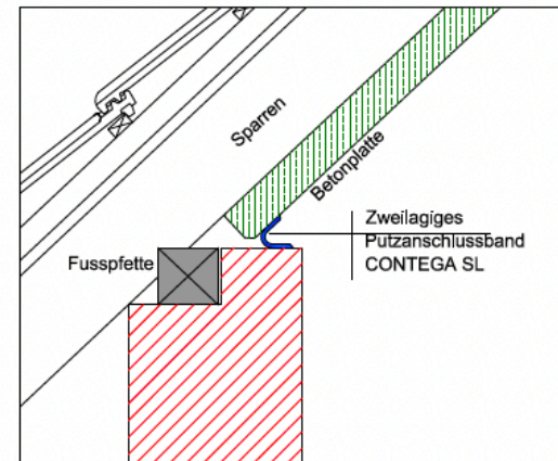
Detail 5 M. 1 : 10
