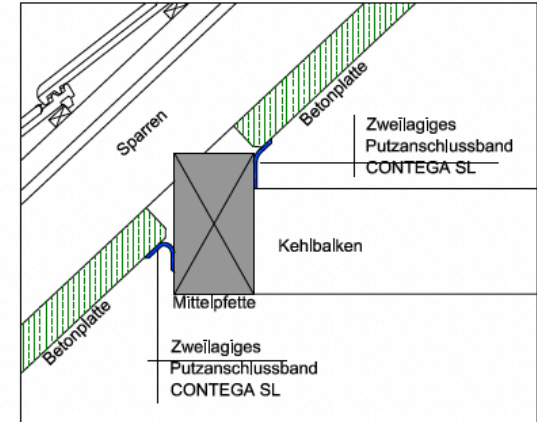
Detail 3 M. 1 : 10
