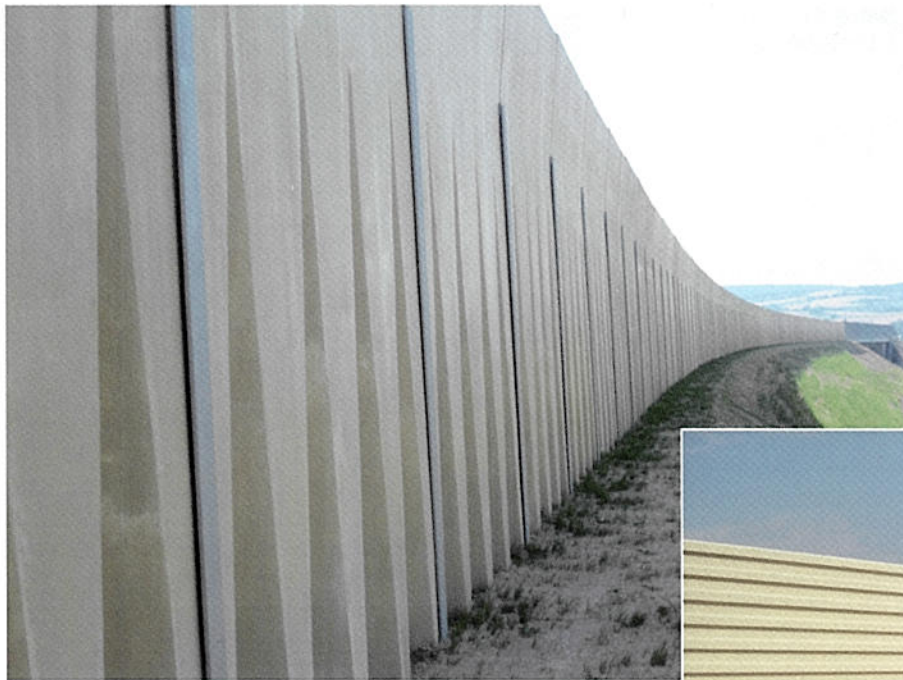
Lärmschutzwände an der A71 Artern
